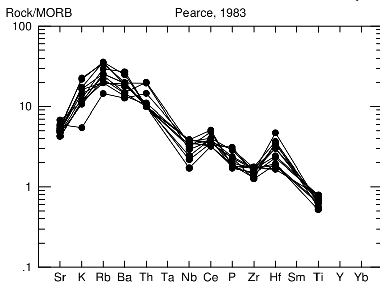
شکل ۷. الگوی فراوانی عناصر ناسازگار بازالت‌های جواهردشت به‌همچنان شده با مقادیر مورب [۵]
