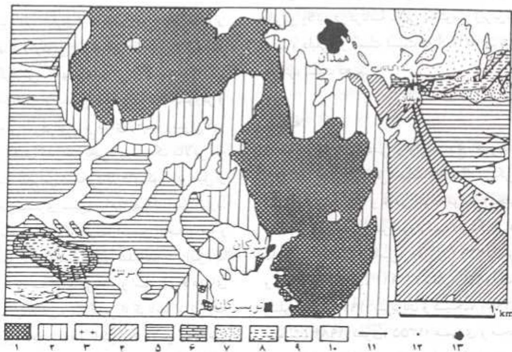
شکل ۱- نقشه زمین‌شناسی منطقه. ۱- نوده گرانیتوئید الوند، ۲- هورنفلس و هورنفلس شیت، ۳- پگماتیت، ۴- انواع شیت، ۵- اسلیت، ۶- آهک‌های ژوراسیک بالایی، ۷- ماسه‌سنگ کرتاسه، ۸- آهک و مارن کرتاسه، ۹- رسوبات میوسن، ۱۰- کواترنری، ۱۱- گل، ۱۲- روستا، ۱۳- شهر. (اقتباس با تغییراتی در چینه‌شناسی از نقشه زمین‌شناسی
