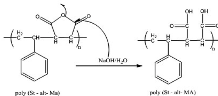
شکل ۱. مکانیسم تبدیل کوپلیمر (استایرن-متناب-مالنیک انیدرید) به کوپلیمر (استایرن-متناب-مالنیک اسید)
