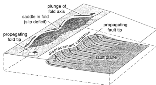
شکل ۸. گسترش جانبی رانندگی زیرسطحی باعث توسعه چین‌خوردگی در پوشش رسوبی زیادی می‌شود. نرخ لغزش متفاوت این گسل، در شدت بالا آمدگی و چین‌خوردگی تاقدیس بالایی آن مؤثر است [۸]
