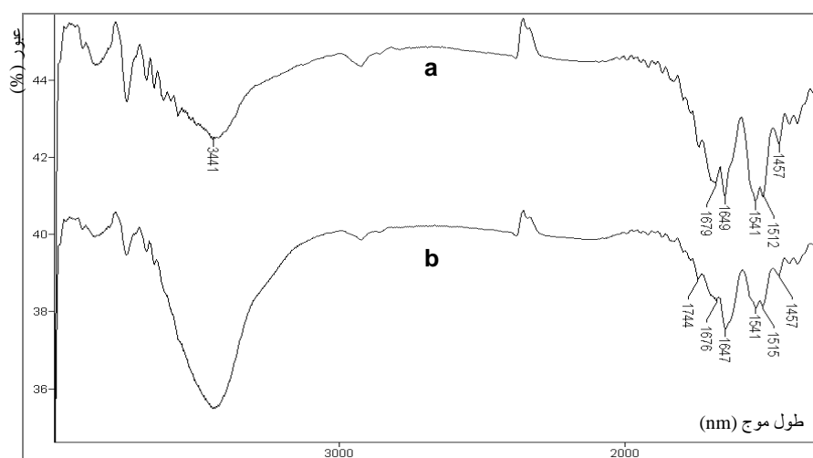
شکل ۵. طیف IR مخلوط آکریل آمید و شبکه‌ساز MBA (a) هیدروژل حاصل از آن‌ها (b)
