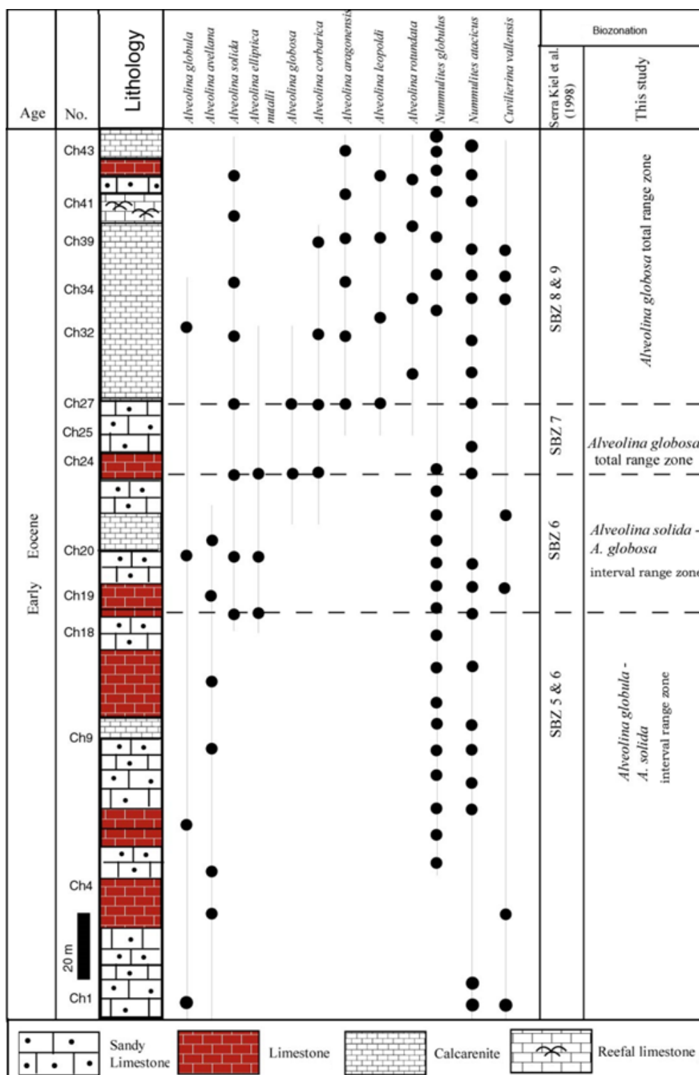
شکل ۲. ستون چینه‌شناسی برش چلونک نشان‌دهنده گسترش چینه‌شناسی فرامینیفرای و بیوزون‌های آلونولین
