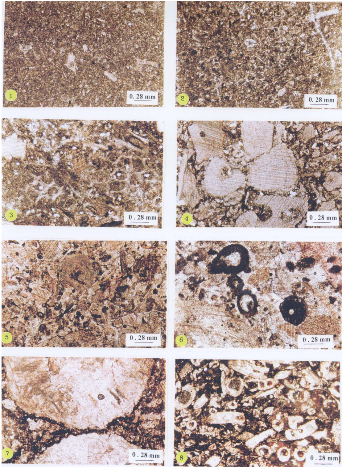
۱- بیوکلست مادستون. ۲- بیوکلست استراکود مادستون / وکستون. ۳- اکینودرم ، بریوزونر بیوکلست وکستون / پکستون . ۴- بیوکلست اکینودرم پکستون. ۵- بیوکلست اکینودرم گرینستون . ۶- میکرو انکوئید ، اکینودرم بیوکلست گرینستون ۷- کورال باندستون . ۸- بیوکلست داسی کلاآسه آ پکستون
