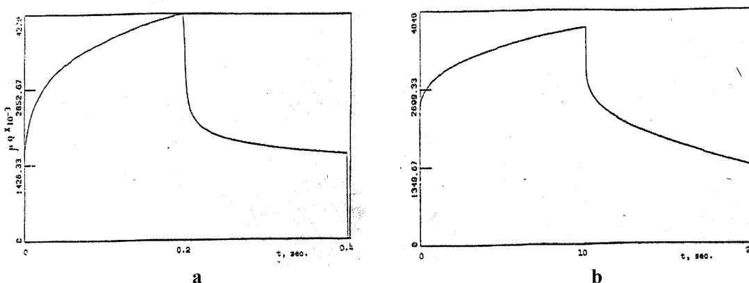
شکل ۴- (a) منحنی کروماتوگرافی الکترودهای نازک طلا 300 \text{ \AA} در الکترولیت 0.1 \text{ M LiClO}_4 ، تغییرات پتانسیل از 0.5 به 0.35 ولت نسبت به SCE (b) منحنی کروماتوگرافی الکترودهای نازک 1000 \text{ \AA} ZnPC در الکترولیت 0.1 \text{ M LiClO}_4 ، تغییرات پتانسیل از 0.5 به 0.35 ولت نسبت به SCE
