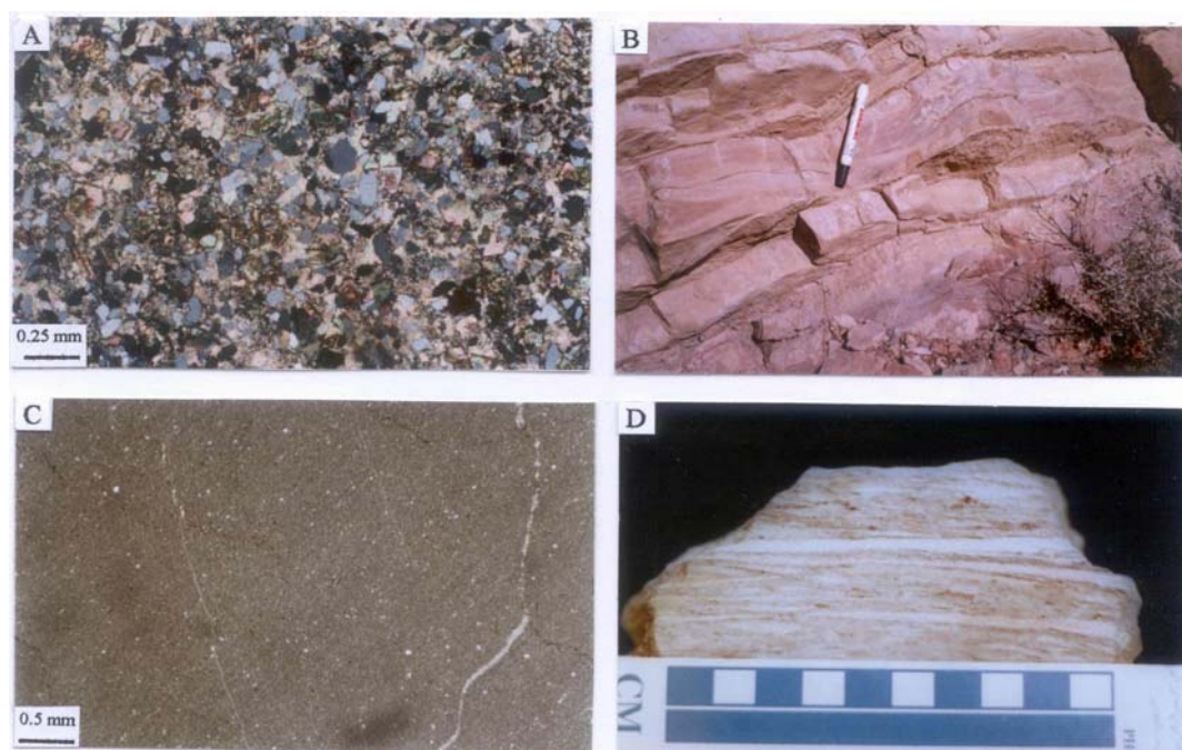
شکل ۶- A- کلکلیتیت مربوط به رخساره P2 (نور پلاریزه). در این تصویر، بلورهای اتومورف دولومیت جانشین خرد شده سنگ‌های آهکی شده‌اند. زمینه سیمان کلسیتی است (نمونه از برش گذار گچال، نور پلاریزه) B- چین‌بندی مورب پشته‌ای (در محل مقیاس) در رخساره طوفانی آواری (نمونه از برش اسلام‌آباد). C- مدستون آهکی لامینه‌دار از زیررخساره Q1. در این تصویر، کوارتزهای آواری در ابعاد سیلیت نیز مشاهده می‌شوند (نمونه از برش اسلام‌آباد) D- نمونه دستی از ژیبس لامینه‌دار در زیررخساره Q3. در این تصویر، هر واحد از خطکش مقیاس برابر یک سانتی‌متر است (نمونه از برش اسلام‌آباد)
