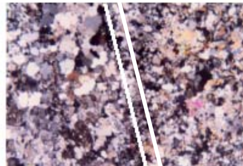
شکل ۱۸. هورنفلس در سمت راست و گرانیت در سمت چپ تصویر قرار دارد ( \times 25.XPL ).
