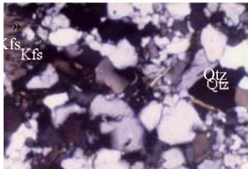
شکل ۱۹. پدیده سیلیسی شدن در هورنفلس‌های دربند شوردر شمال گلپایگان ( \times 100.XPL ).
