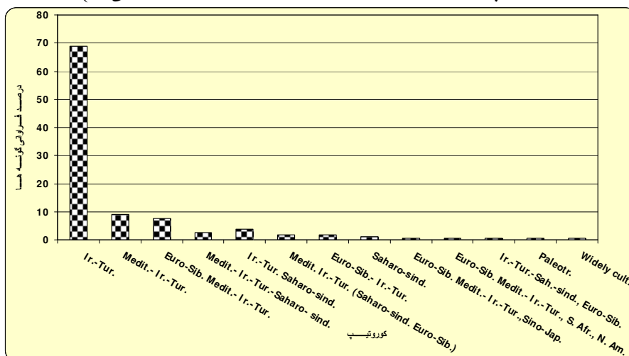
شکل ۵. درصد فراوانی پراکنش جغرافیایی گونه‌های گیاهی ارتفاعات کلات_ زیرجان گناباد (Euro-Sib.، Ir.-Tur.، Meditrane، Paleotr.، N. Am.، S. Afr.، Sino-Jap.، Saharo-sind.، Euro-Sib.، Ir.-Tur.، S. Afr.، N. Am.، اروپا-سیبری، صحرا-سندی، سینو-ژاپنی، آفریقای جنوبی، آمریکای شمالی، پالئوتروپیک است)
