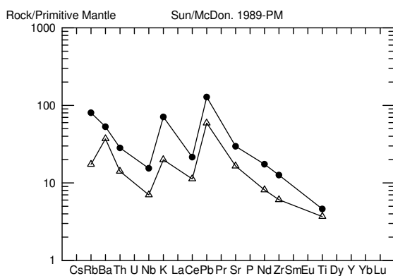
شکل ۹. مقایسه الگوی میانگین عناصر ناسازگار بازالت‌های جواهر دشت با مقادیر پوسته زیرین [۱۵] Δ پوسته زیرین ● بازالت‌های جواهر دشت
