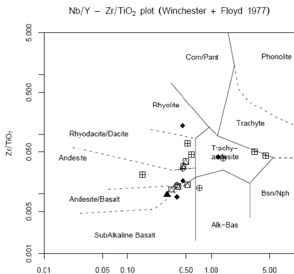
شکل ۶. نمودار Zr/TiO_2 در مقابل Nb/Y [۱۱]، بر مبنای این نمودار سنگ‌های آتشفشانی منطقه آشتیان در قلمرو بازالت ساب آلکان، آندزیت بازالتی، آندزیت، تراکی آندزیت، داسیت، ریوداسیت و ریولیت قرار گرفته‌اند
