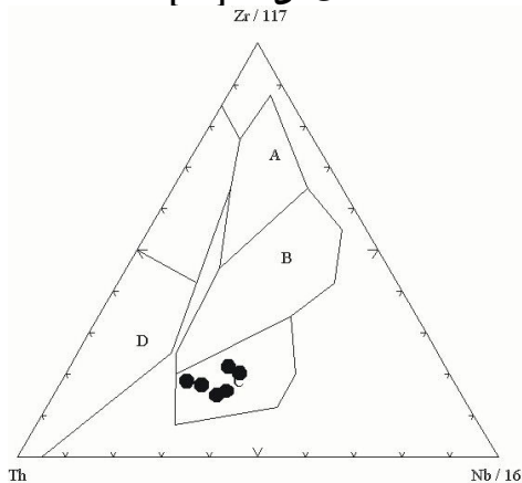
شکل ۱۱. نمودار متمایز کننده محیط تکتونیکی بر اساس عناصر غیرمتحرک. محدوده‌ها نماینده A: مورب نوع N، محدوده B: مورب نوع E و بازالت‌های تولنییتی درون صفحه‌ای، محدوده C: بازالت‌های درون صفحه‌ای و محدوده D: بازالت‌های قوس آتشفشانی‌اند [۱۲]
