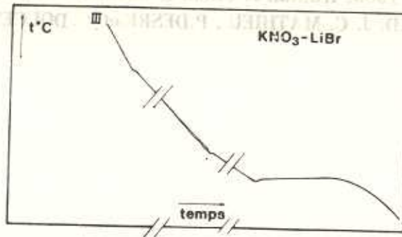
شکل ۴ منحنیهای دما - زمان در غلظتهای برای سیستم نیترات پتاسیم برمید لیتم
