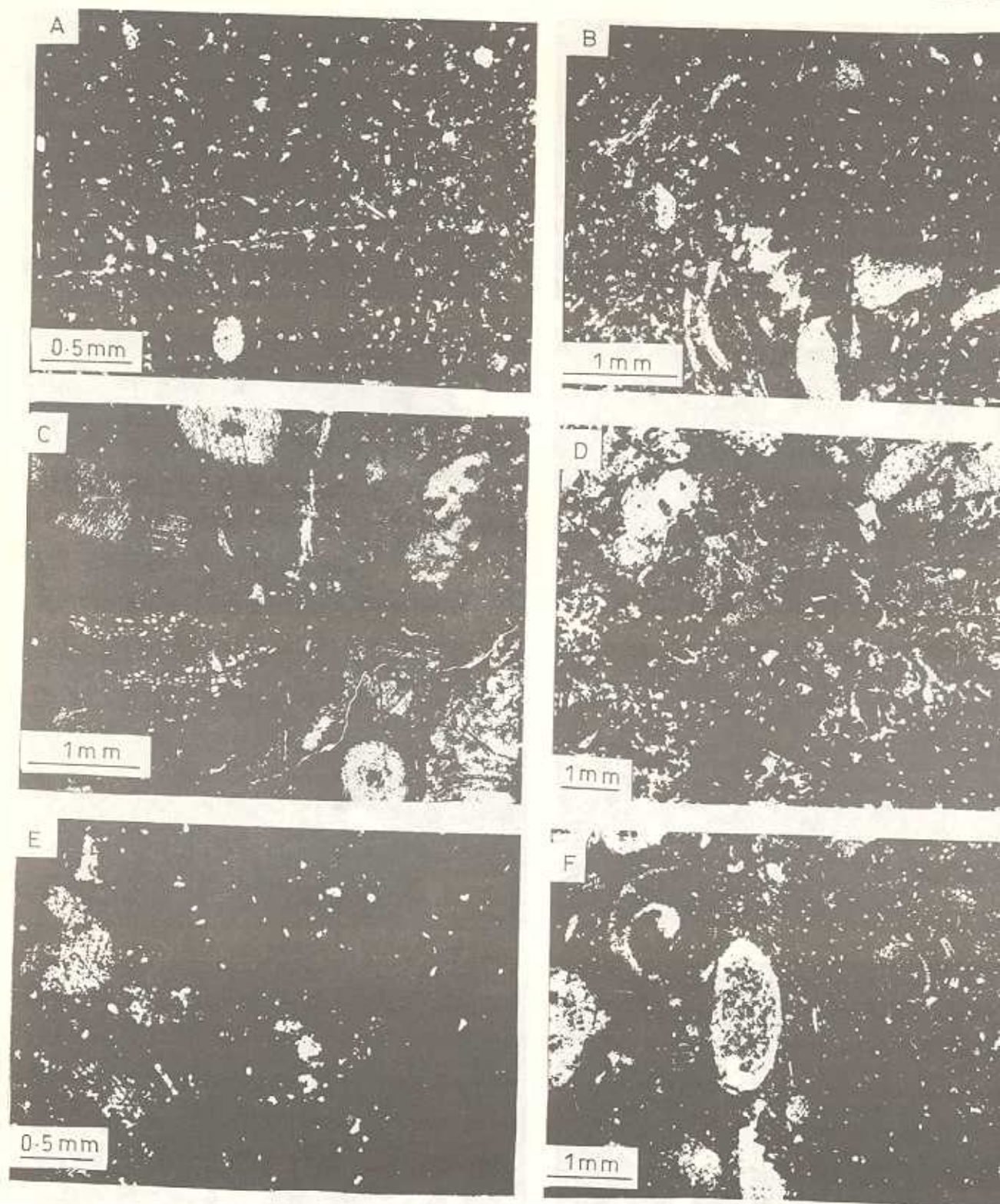
شکل ۲: میکروفاسیس های دریای باز (A-D) و میکروفاسیس های بخش رو به دریای لاگون (E-F) در سازند مبارک پشت سد بیوکلاستی
