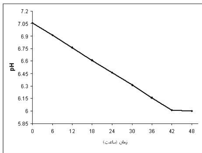
شکل ۳. کاهش pH در اثر فعالیت غشای ارغوانی خالص سازی شده
