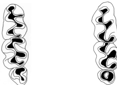
شکل ۵. طرح دندانی هامستر دم‌دراز از منطقه حفاظت شده گنو (۶x)
