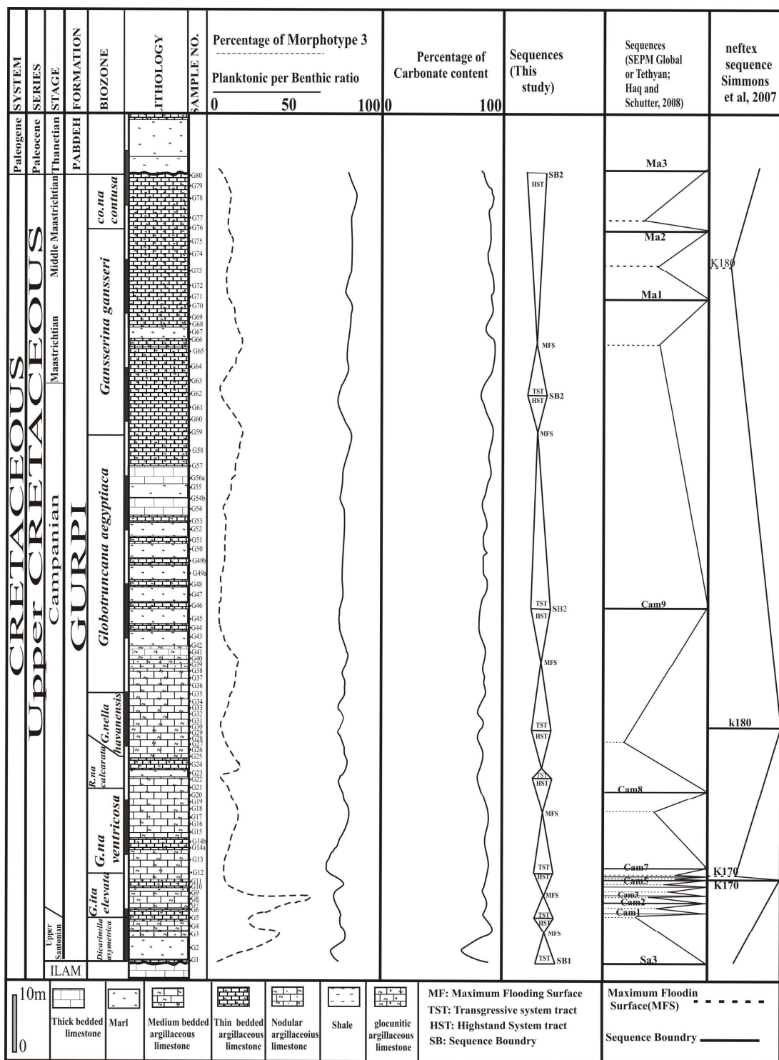
شکل ۳. تطابق سکانس‌های ارائه شده برای سازند گورپی در جنوب غرب فیروزآباد با سکانس‌های جهانی [۲۷] حق و شاتر (۲۰۰۸)، و سکانس‌های ارائه شده برای ورقه عربی [۲۷] سیمونز و همکاران (۲۰۰۷)
