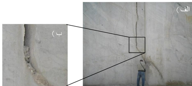
شکل ۶. الف) تصویر درز J7 که با درز پایینی خود ساختار قلاب‌شدگی را نشان می‌دهد. این ساختار داخل محدوده مستطیلی و با پیکان قرمز رنگ مشخص شده است (دید به سمت جنوب باختر) (ب) نمای نزدیک از ساختار قلاب‌شدگی
