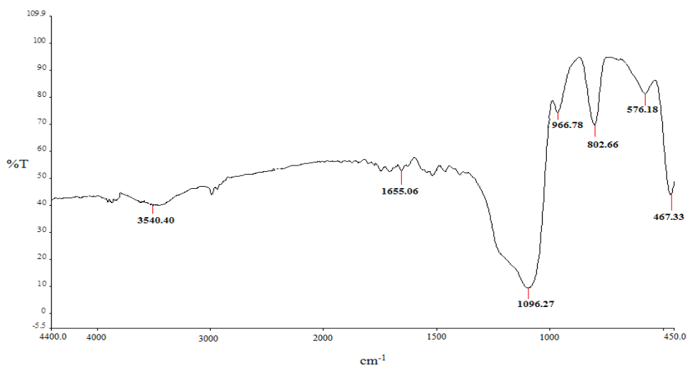
شکل ۴. طیف FTIR نانوذرات هسته-پوسته Fe 3 O 4 /SiO 2
