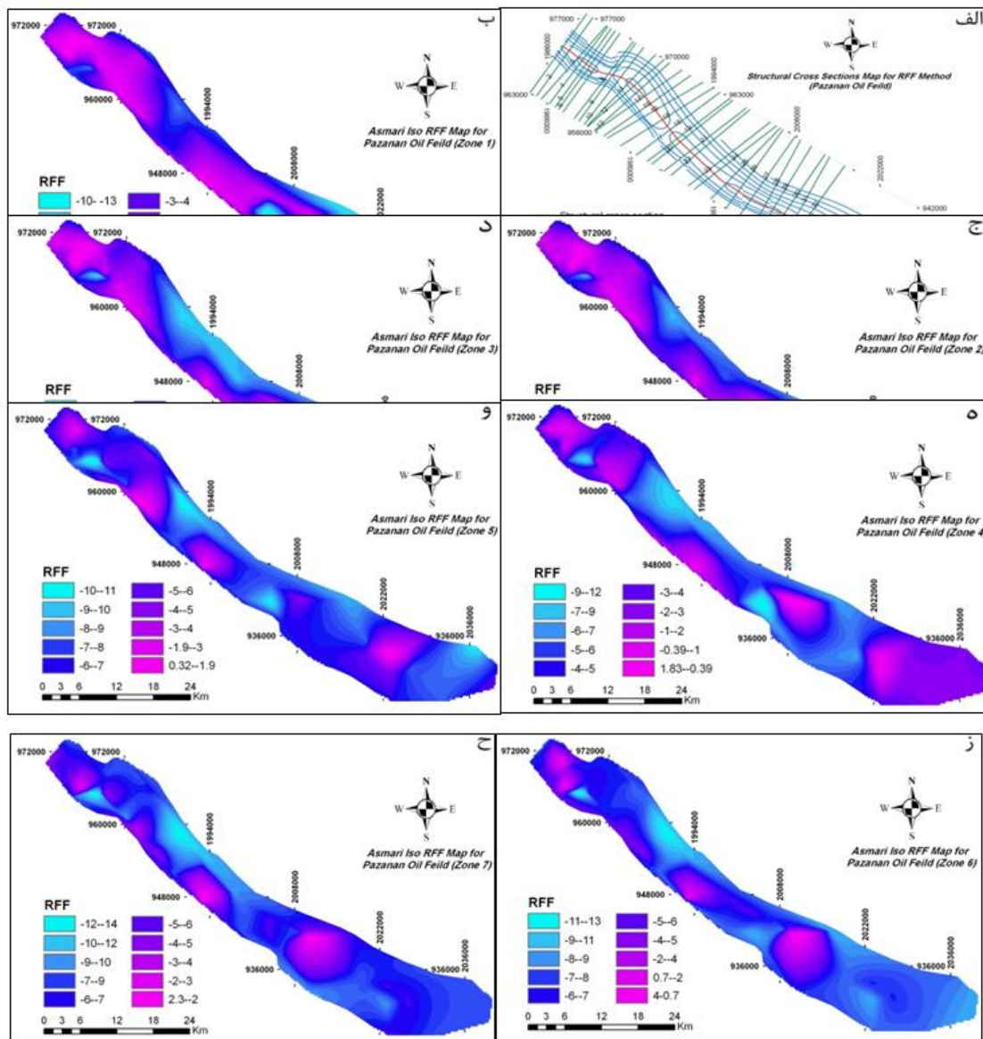
شکل ۶. الف) موقعیت برش‌های عرضی تهیه شده بر روی سرسازند آسماری میدان نفتی پازنان برای به‌کارگیری روش RFF. ب تا ح) به‌ترتیب نقشه‌های ه م RFF برای سرسازند آسماری، عمق منطبق بر میانه پهنه‌های یک، دو، سه و چهار و پنج و شش و هفت سازند آسماری (مناطق قرمز رنگ نواحی دارای حداکثر تراکم شکستگی را نشان می‌دهند)
