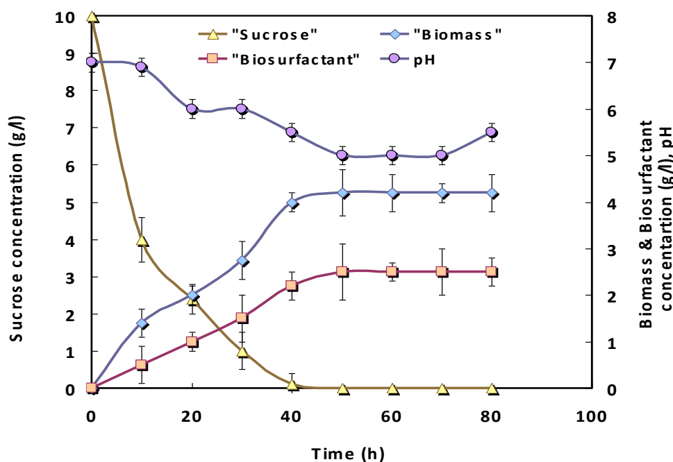
شکل ۲. نمودار رشد سلولی، تولید بیوسورفکتانت، مصرف ساکاروز، \text{pH} تحت شرایط بهینه ( 37^\circ\text{C} و 300 \text{ rpm} و 1/5 \text{ vvm} ) در بیوراکتور طراحی شده
