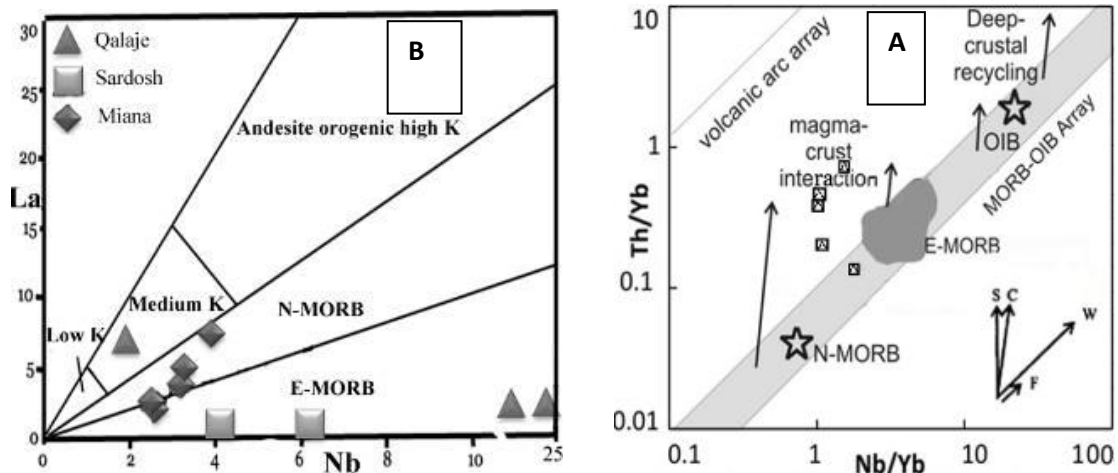
شکل ۹. A) نمودار La/Nb [۲۷]، پراکندگی نمونه‌های میانه و نسل در محدوده بین E-MORB و N-MORB با روند به سمت N-MORB است. دو نمونه از قه‌لاجی و نمونه‌های سردوش در محدوده E-MORB قرار گرفته‌اند که گویای منشأ تهی‌شده‌تر برای این توده‌ها هستند. B) نمودار Ta/Yb-Ta/Yb [۲۸]، برای نمونه‌های میانه نشان می‌دهد که گابروها در جای‌گاه‌های پراکنده‌ای از گوشته تهی‌شده به ماگمای کالک‌الکالن قرار دارد. بردارهای تغییرات شیمیایی ناشی از تبلور تفریقی F، اثرات منبع W، آغستگی پوسته‌ای C و فرورانش S را نشان می‌دهد. با توجه به بردارها تغییرات در بازالت‌ها ناشی از منشأ (W) و گابروها متأثر از فرورانش (S) هستند.
