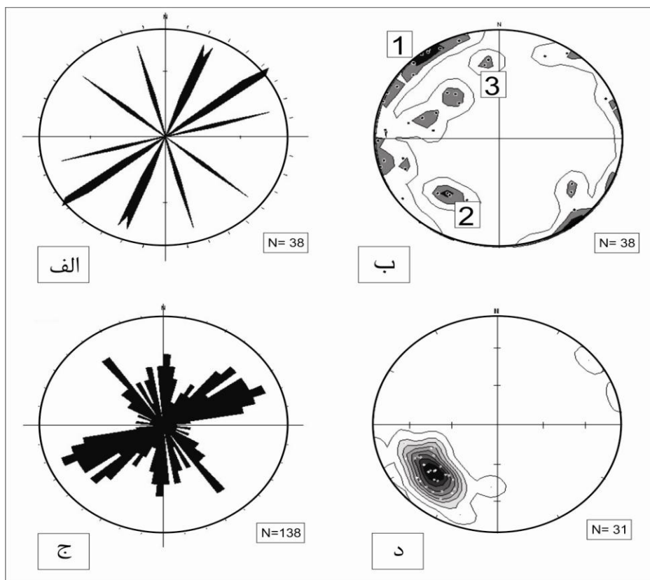
شکل ۳. الف) پراکندگی آماری گسل‌های منطقه بر روی نمودار گلسرخ، ب) پراکندگی آماری گسل‌های منطقه روی نمودار استریونت هم مساحت، شماره ۱، ۲ و ۳ به ترتیب نقاط تجمع بیش‌ترین پراکندگی و سامانه‌های مختلف گسلی مطالعه شده را نشان می‌دهد، ج) نمودار گلسرخ حداکثر درزه و شکستگی‌های موجود در سنگ‌های منطقه، د) نمودار استریونتی هم مساحت شیستوزیته‌های برداشت شده سنگ‌های منطقه
