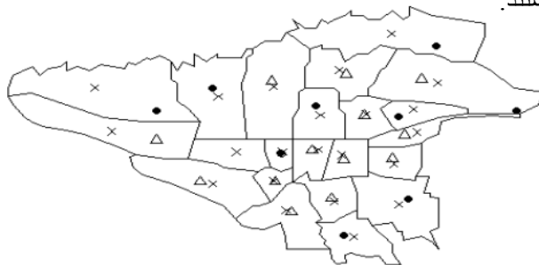
شکل ۵. موقعیت ایستگاه‌های مانیتورینگ (●)، نقاط نمونه‌گیری (×) و ایستگاه‌های فاقد مشاهده (Δ)
