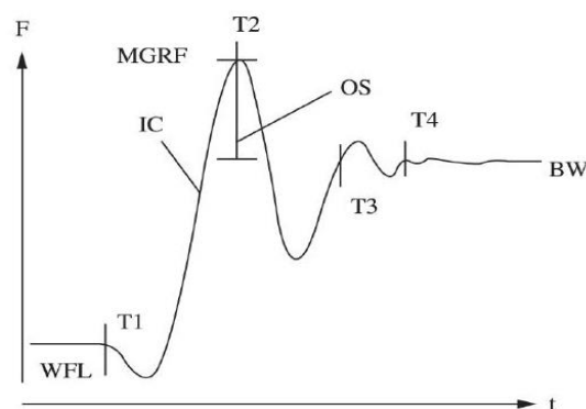
شکل ۱. نمودار مراحل حرکت نشست و برخاست به ۳ مرحله تقسیم‌بندی شده است. مرحله آماده‌سازی (T1-T2) مرحله برخاستن (T2-T3) مرحله ثبات (T3-T4) BW^2 وزن بدن، MGRF (حداکثر نیروی واکنش زمین)، OS^3 (میزان خطا)، IC^4 (شیب)، WFL^5 (وزن کف پا/پا) مرحله برخاستن، T1^6 (شروع حرکت)، T2^7 (نشسته)، T3^8 (برخاستن)، T4^9 (پایان حرکت) (۳۰)
