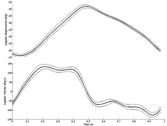
نمودار ۱: میانگین کل جابجایی و سرعت زاویه ای مفصل ران در سی سیکل رکاب زدن
