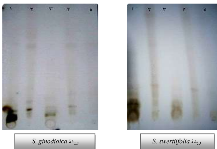
شکل ۶- کروماتوگرام مربوط به فرکشن‌های مختلف استخراج ساپونین از ریشه‌های Silene ginodioica و Silene swertiifolia .
