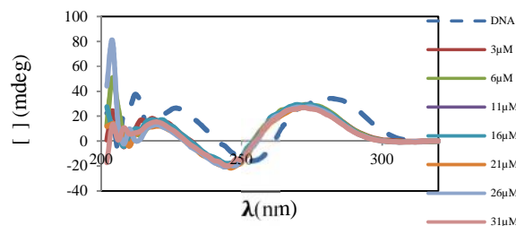
شکل ۸- طیف CD ساختار DNA در حضور غلظت‌های (۳، ۰، ۶، ۱۱، ۱۶، ۲۱، ۲۶، ۳۱ میکرومولار) نانو ذرات اکسید روی.
