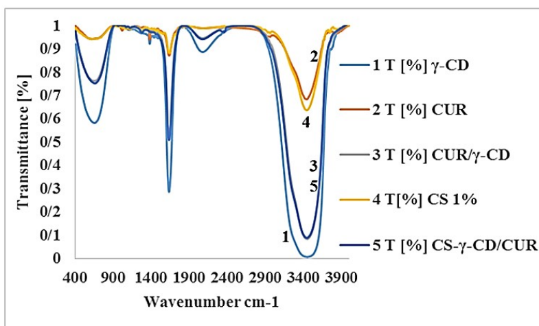
شکل ۴- طیف‌های FTIR برای \gamma -CD خالص، CUR آزاد، کمپلکس CUR/ \gamma -CD، CS خالص و کمپلکس اصلاح شده CS/ \gamma -CD-CUR. Figure 4. FTIR spectra for pure \gamma -CD, free CUR, pure CUR/ \gamma -CD complex, pure CS1% and pure CS CUR/ \gamma -CD-CS modified complex.
