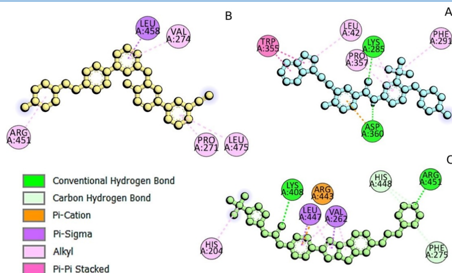
شکل ۲- برهمکنش آنزیم UGT1A3 با A) پناآتینیب B) تپوتینیب C) کوئیزاتینیب. ساختار لیگاندها در وسط هر تصویر و اسید آمینه‌های آنزیم در اطراف آن نشان داده شده است. برهمکنش‌ها با نرم افزار دیسکاویری استودیو بررسی و تصویر آن ذخیره شد.
