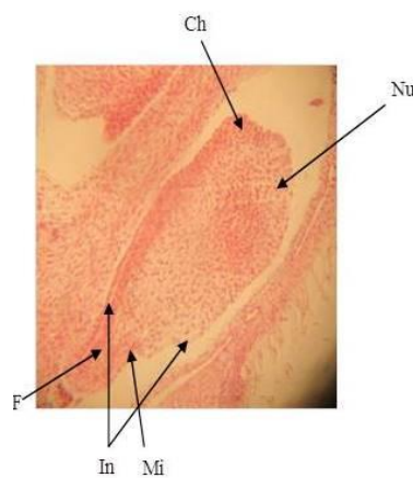
شکل ۱۳- تخمک بالغ تک پوسته‌ای به همراه اجزای تشکیل دهنده آن؛ Ch: بن یا شالاز، Nu: خورش، In: پوسته تخمک، Mi: سفت، F: سوسپانوسور یا بند. بزرگنمایی ۷۶۸ x.
