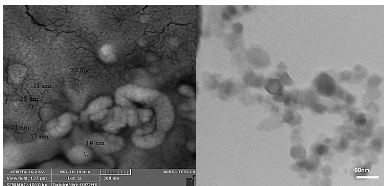
شکل ۱- تصاویر نانوذره سلنیوم برحسب نانومتر (nm)، SEM (راست) و TEM (چپ). Figure 1. SEM (right) and TEM (left) of selenium nanoparticles.
