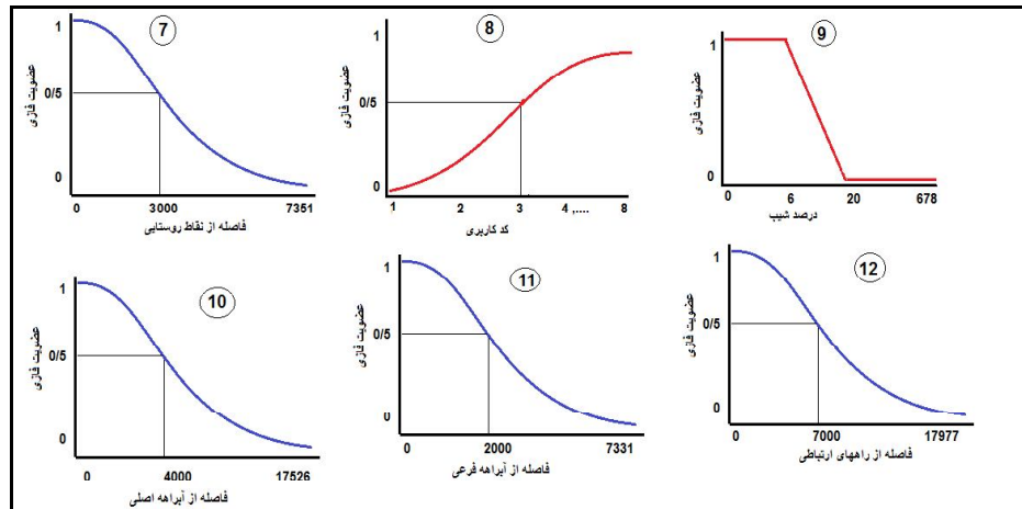
شکل شماره (۵): توابع فازی سازی معیارهای (۷) فاصله از نقاط روستایی (۸) کاربری اراضی (۹) شیب (۱۰) فاصله از آبراه اصلی (۱۱) فاصله از آبراه فرعی (۱۲) فاصله از راههای ارتباطی
