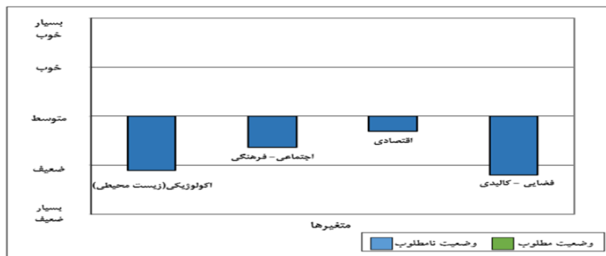
شکل ۴. نمودار شاخص‌های توسعه اکوتوریسم
