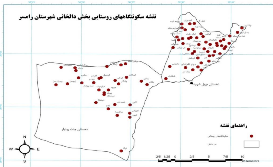
شکل ۳. نقشه پراکنش سکونتگاه‌های روستایی بخش دالخانای به تفکیک دهستان
